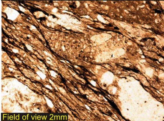
Roseland breccia ppl
