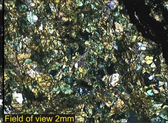
Skarn xpl
