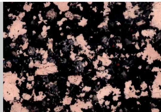
Luxullianite xpl
