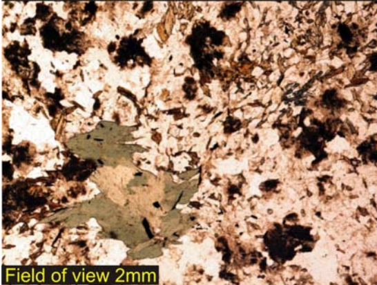
Gneiss ppl
