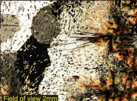
Luxullianite xpl
