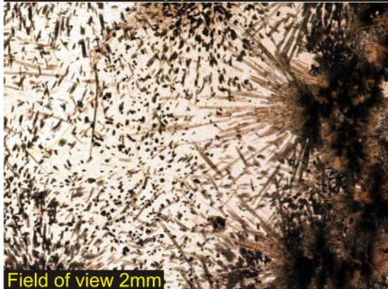
Luxullianite ppl
